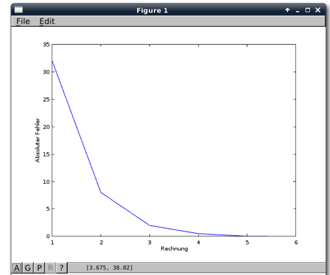
Der Plot des absoluten Fehlers. 🔍
